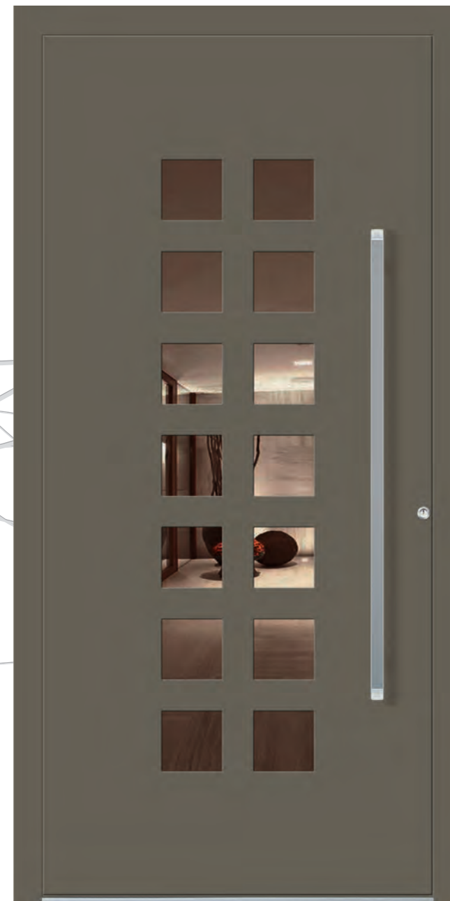
Modell TR98E Farbe RAL 7039 Verglasung FLOAT Griff KPR 115h Rosette RMM
