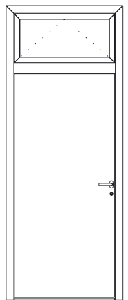
Haustür DIN rechts einflügelig mit Kipp-Oberlicht Door - single, right with Transom light tilt opening
